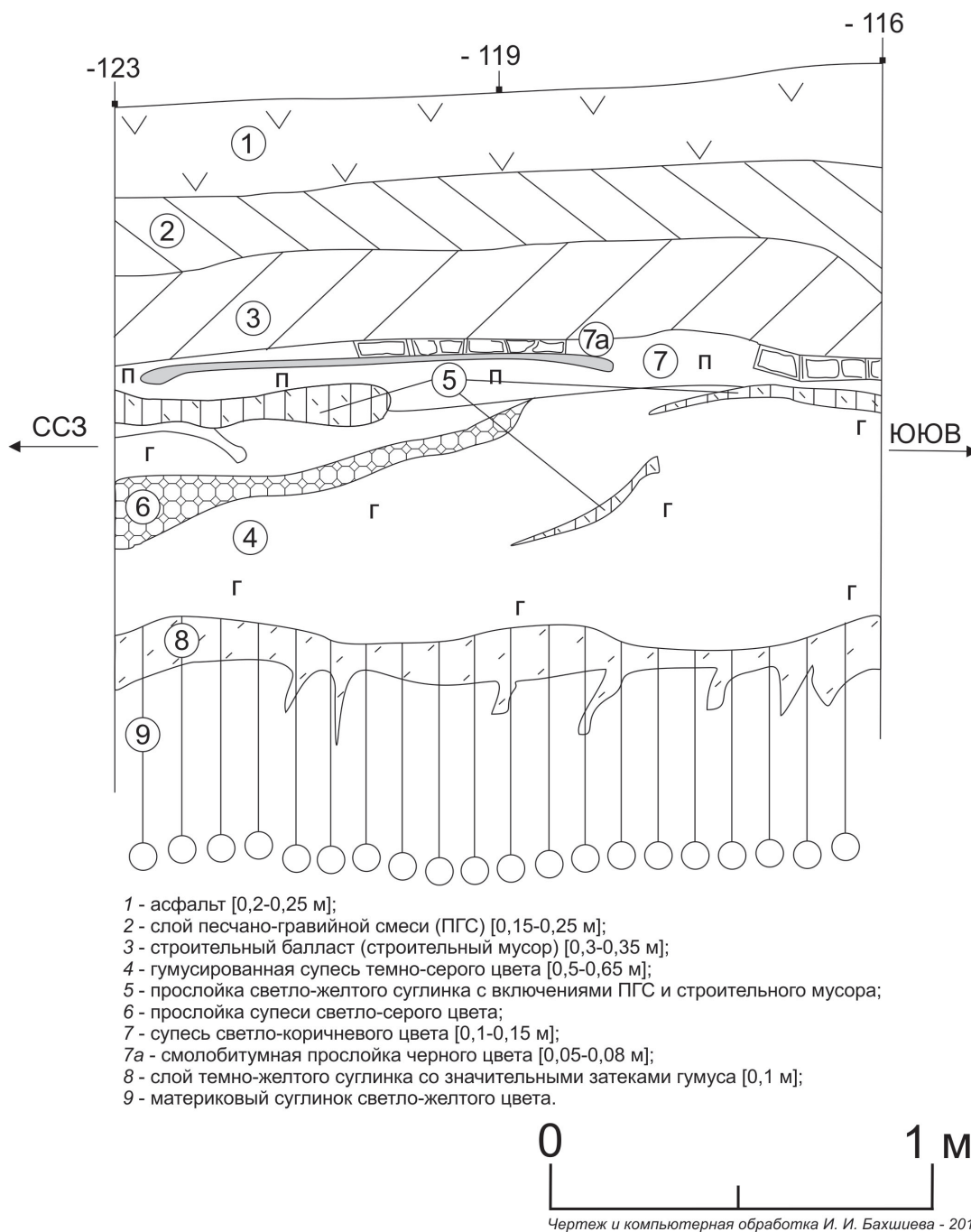
Рис. 4. Республика Башкортостан, город Уфа, ул. Театральная, 3. Локальный стратиграфический разрез восточного борта строительного котлована
