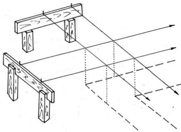
Рис. 2 Закрепление осей строящегося здания
