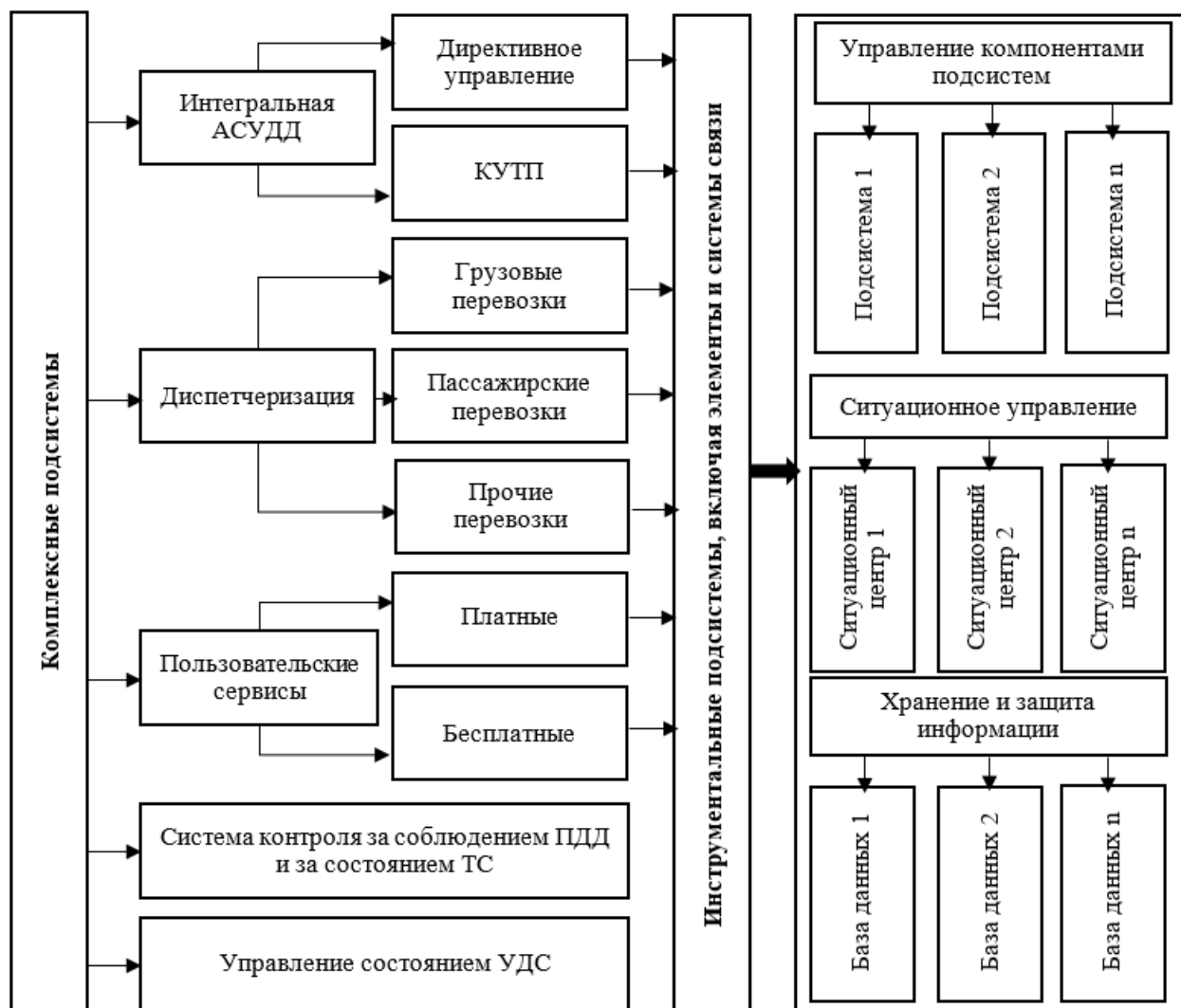
Рис. 3 Физическая архитектура ИТС РФ
