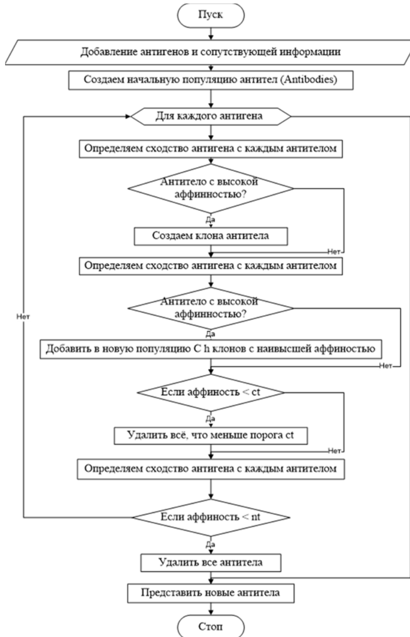
Рис. 3 Алгоритм реализации
