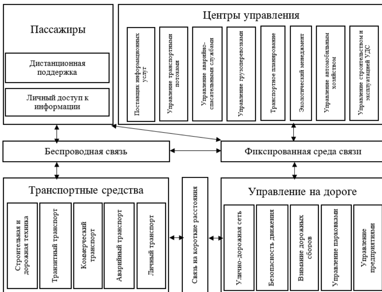
Рис. 1 Физическая архитектура ИТС США
