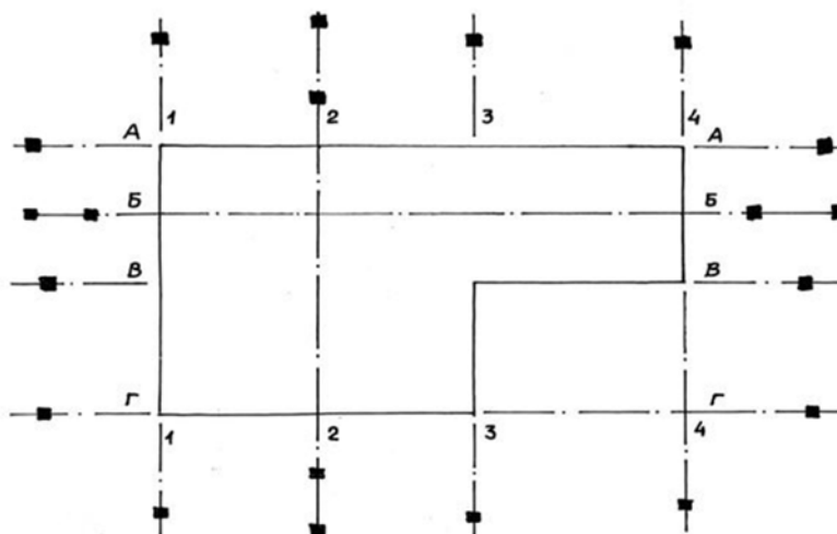
Рис. 1 Разбивка фундамента
