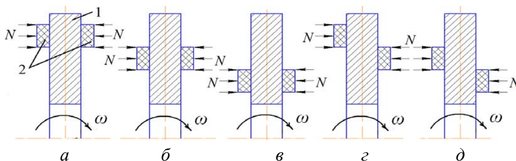
Рис. 2 Схемы фрикционного взаимодействия пар трения дисково-колодочного тормоза со смещением накладок по отношению к боковым поверхностям диска: а, б, в – параллельном; г, д – последовательном; 1 – тормозной диск; 2 – фрикционные накладки; N – усилие нажатия; \omega – угловая скорость диска
