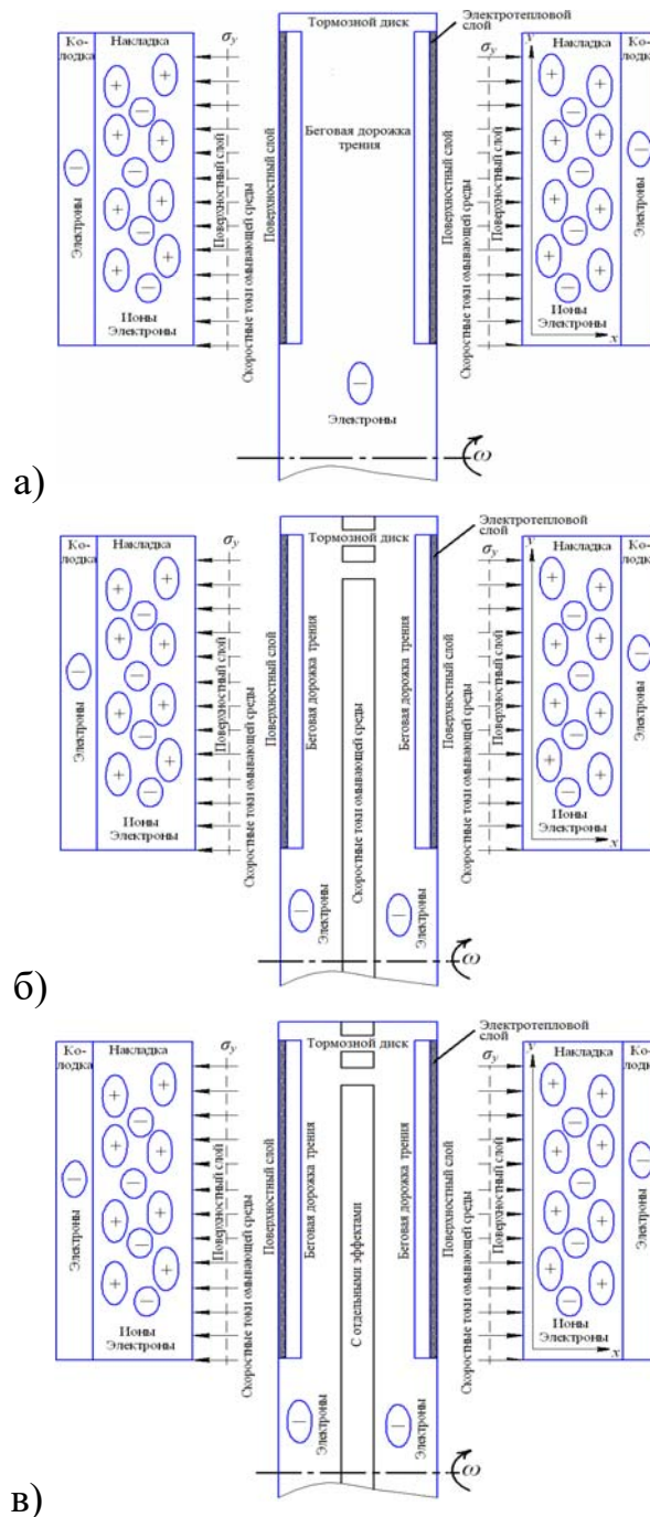
Рис. 1 Электронно-ионная схема трибосистемы дисково-колодочного тормоза с дисками различного типа: а – сплошным; б – самовентилируемым; в – с отдельными эффектами: кондуктивным, многоструйного эжектора, вихревого и тепловой трубы
